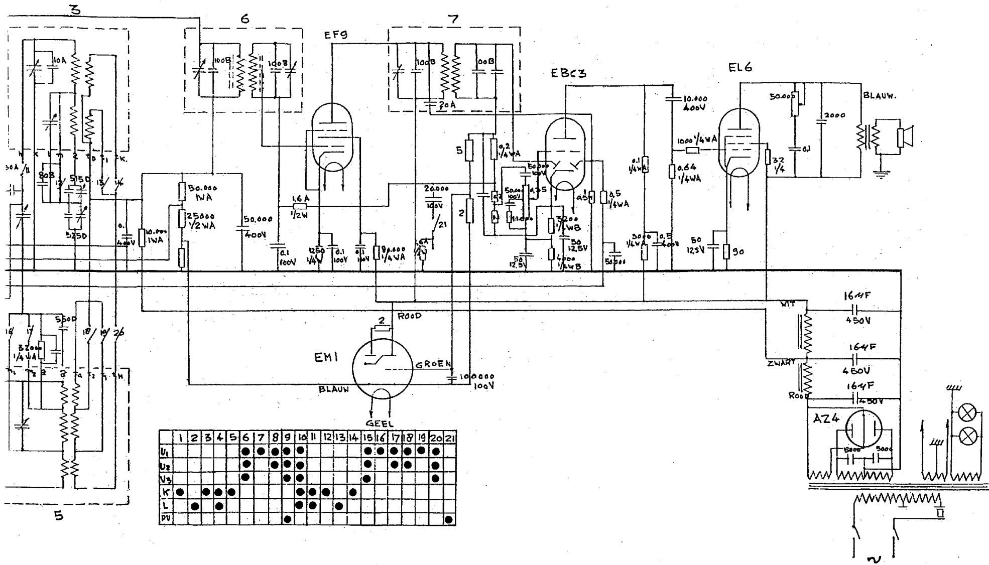
SCHEMA APP. 178 GET. AP , GEZ.
